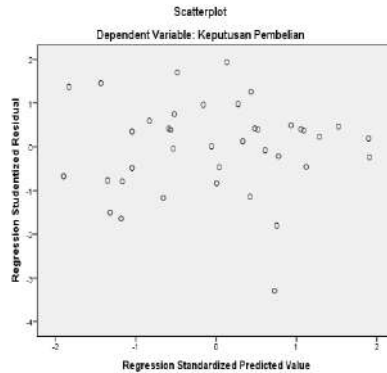
Gambar 2. Uji Heterokedastisitas
